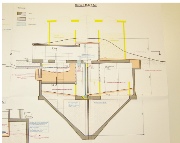
Projektplan für den Umbau der ARA
